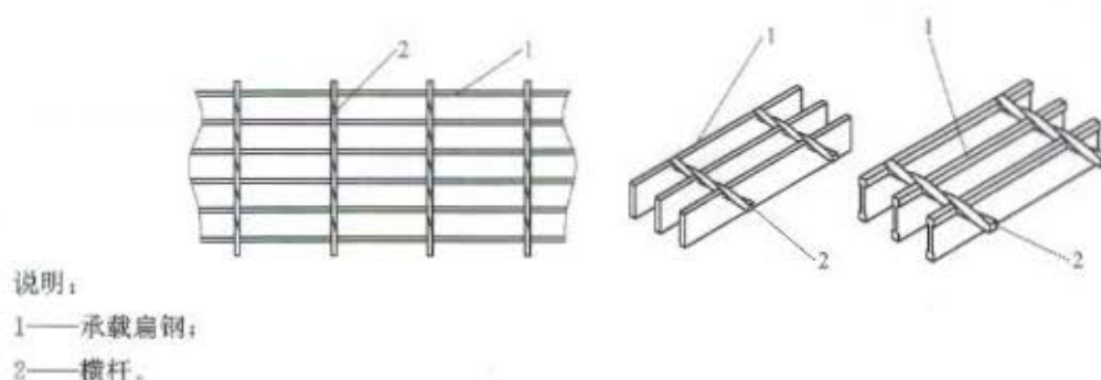
图1 压焊钢格板
