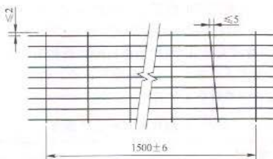
图 5 横杆间距和垂直偏差
