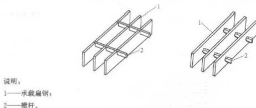
图2 压锁钢格板
