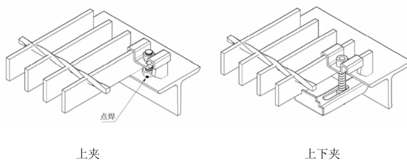
图B.5 钢格板的安装夹固定
